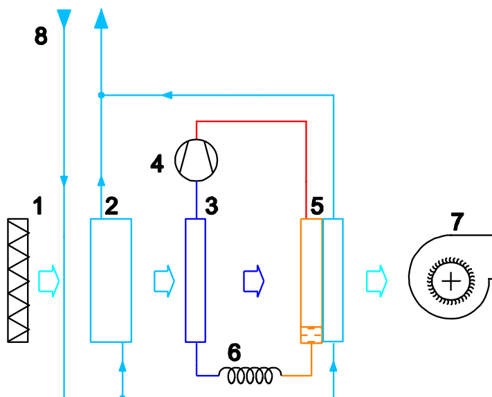
Fig. 1 Schema del deumidificatore DEW 26-S
