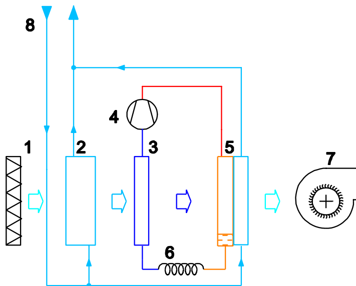
Fig. 1 Schema del deumidificatore DCS26BD
