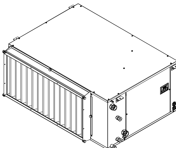
Fig. 1: Deumidificatore da controsoffitto, cod. 2013.00.02 (DEW CAP 750B) e cod. 2015.00.02 (DEW CAP 1000B)
