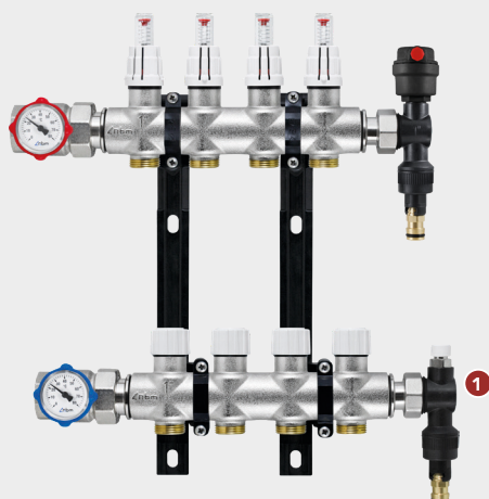
Kit collettori compatti in ottone nichelato
