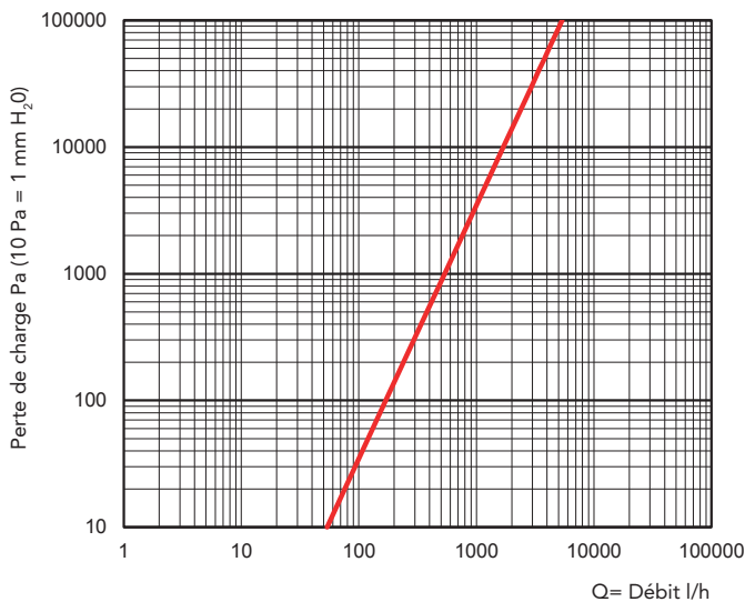
Diagramme pertes de charge
