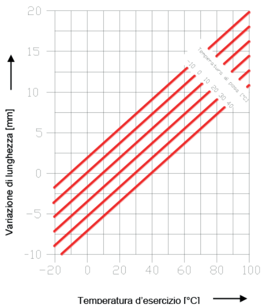
Grafico 3 Dilatazione di 1 m di tubo KILMA-FLEX 4 FIN
