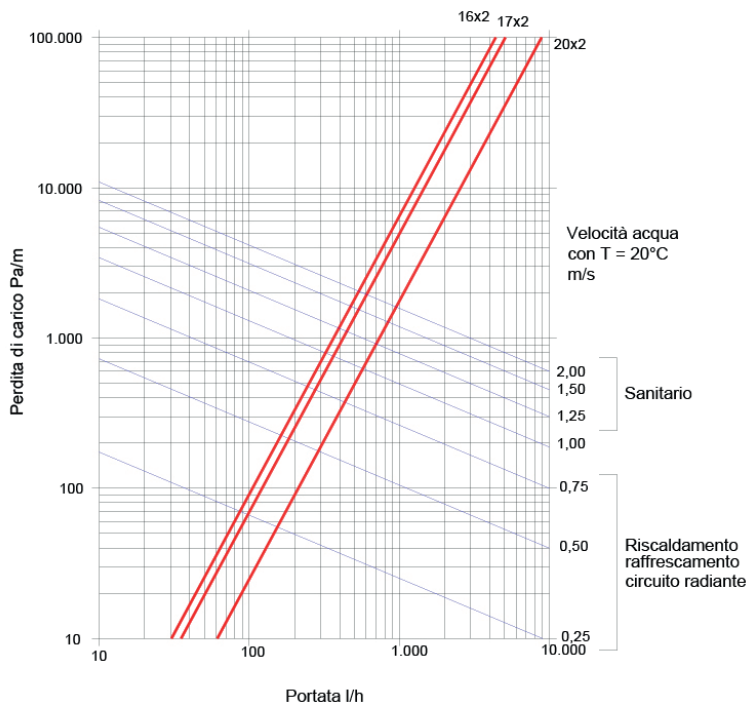
Grafico 4 Perdite di carico nel tubo KILMA-FLEX 4 FIN
