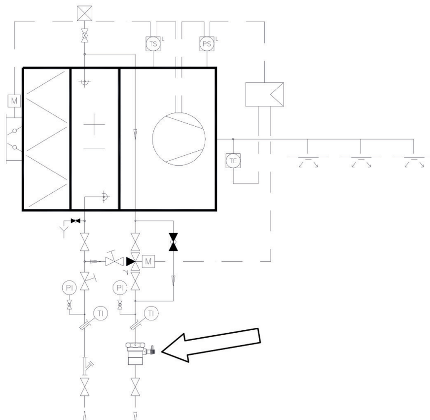
FIGURA 5 Misurazione della portata per taratura gruppi di termoregolazione su centrali di trattamento aria.
