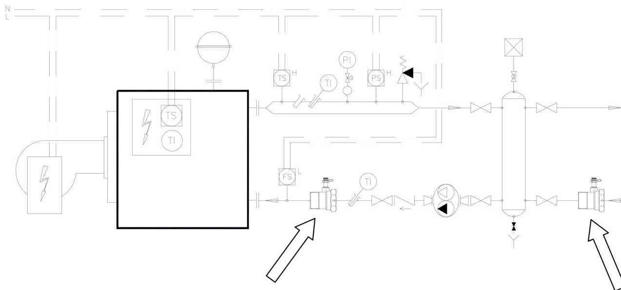
FIGURA 6 Misurazione della portata per le verifiche prestazionali di una Centrale termica.
