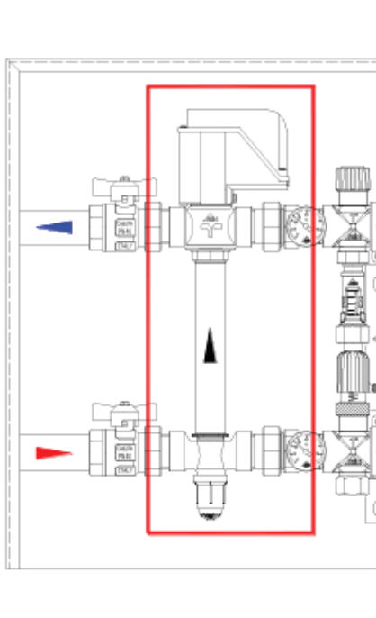
Composizione kit collettore con valvola di zona: L1 + 110 mm
