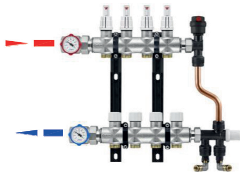
Corretta installazione del collettore con flussometro
