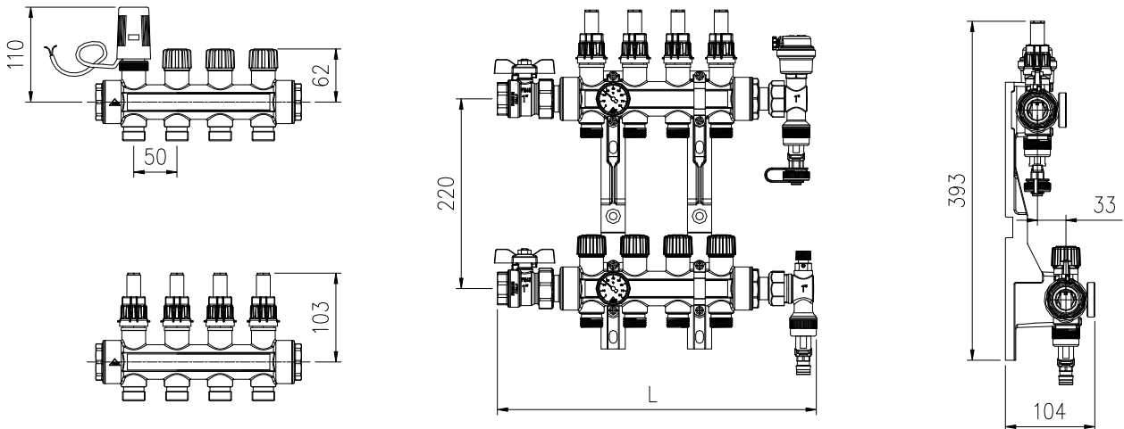
Afmetingen verdeler
