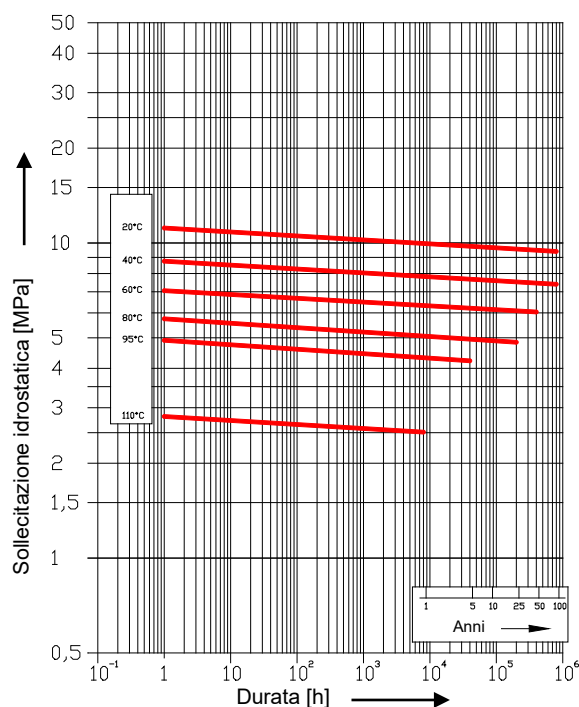
Grafico 1 - Diagramma realizzato secondo EN ISO 15875-2
