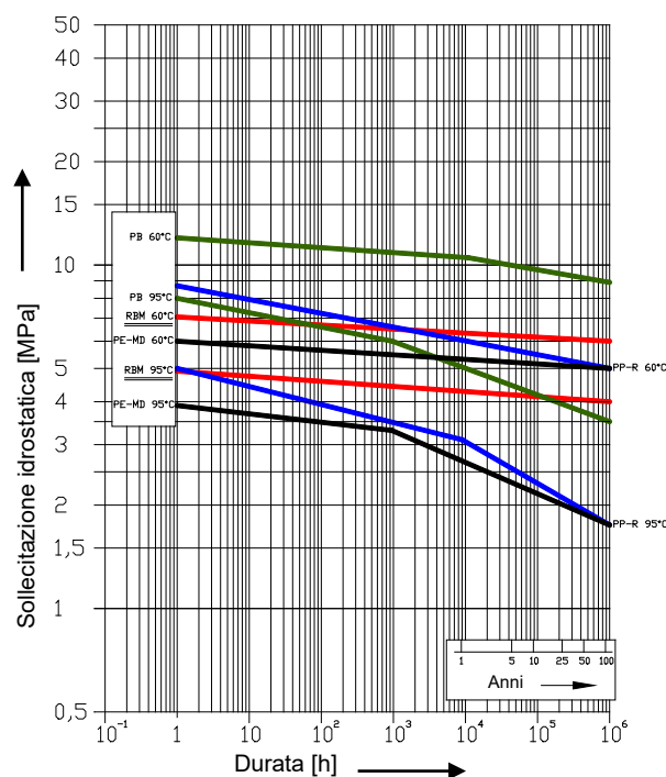
Grafico 2 - Curve di regressione a confronto: PE-Xc, PP-R, PB, PE-MD
