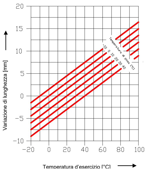
Grafico 3 – Dilatazione di 1 m di tubo RBM KILMA-FLEX PE-Xc
